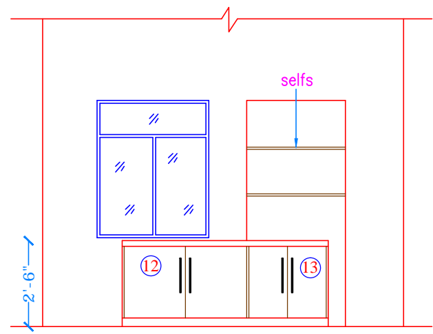
ELEVATION "C"
